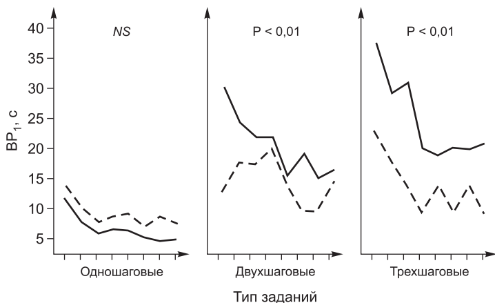
Рис. 1.11. Время реакции импульсивных (на рисунке их графики обозначены пунктирной линией) и рефлексивных (их график обозначен сплошной линией) испытуемых при решении задач на аналогии (Т. Jurack, 1982). Буквы «NS» указывают на незначимость различий
